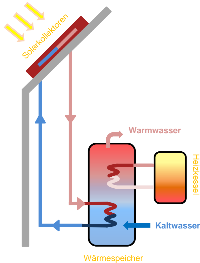
Schematische Darstellung der Funktionsweise einer solarthermischen Anlage (eigene Darstellung)
